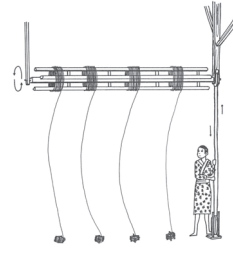
羽1_G008_140図-イトアゲルマ・アゲワク組合せ図
